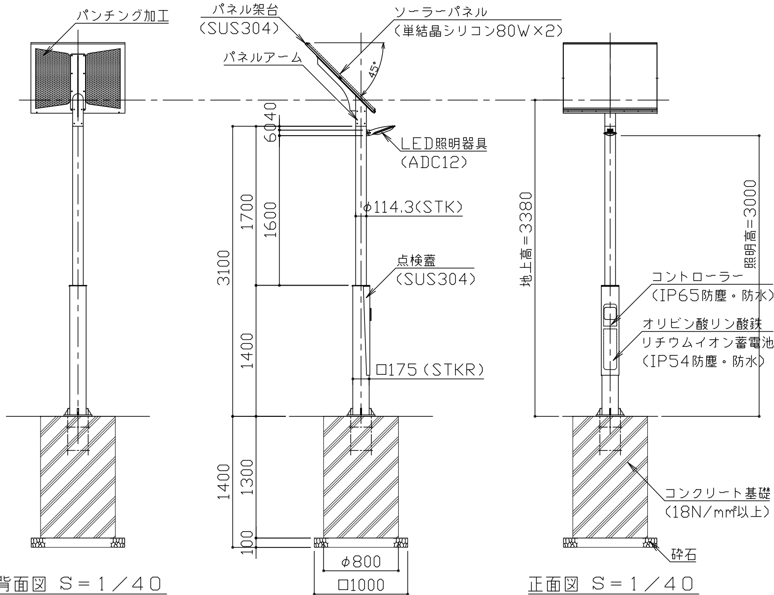
側面図 S = 1 / 40
