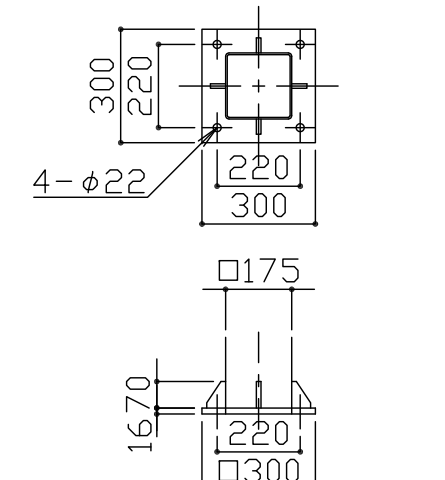
ベースプレート詳細図 S = 1 / 20
