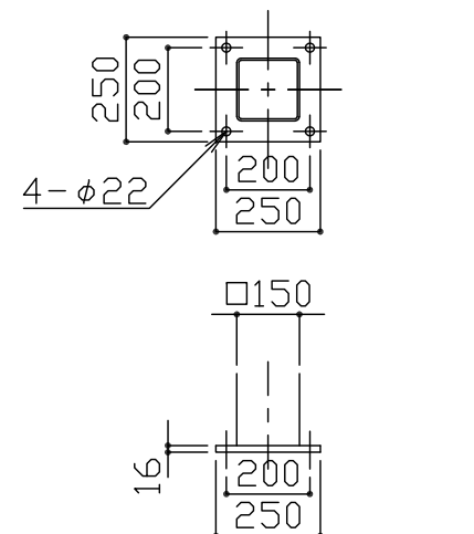
ベースプレート詳細図 S = 1 / 20
