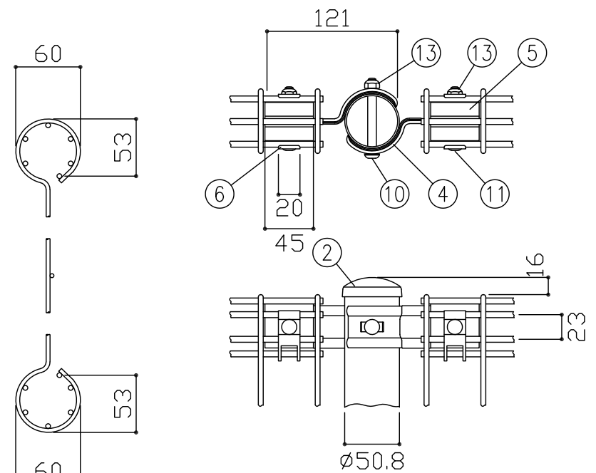
A部詳細図 S = 1 / 5
