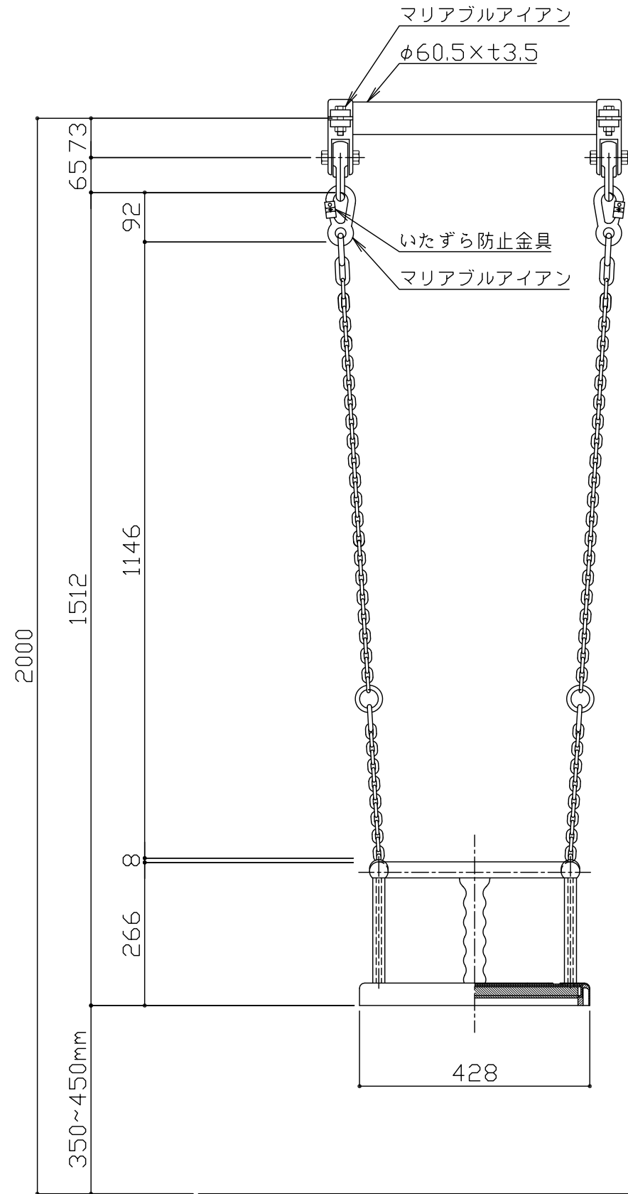
立面図 S = 1 / 10
