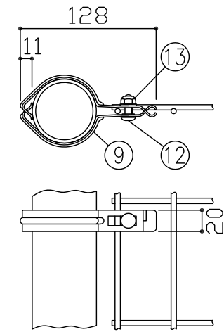
D部詳細図 S = 1 / 5
