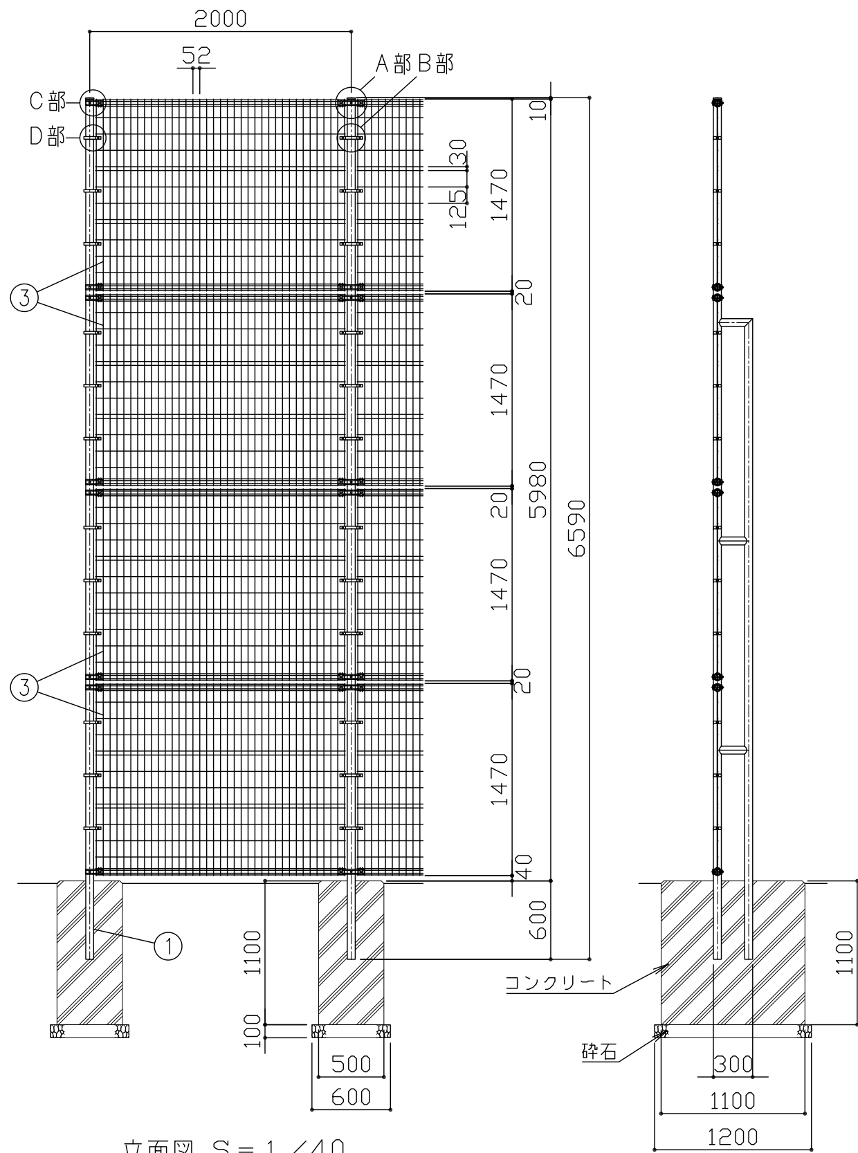
立面図 S = 1 / 40
