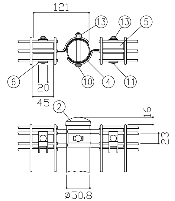
A部詳細図 S = 1 / 5
