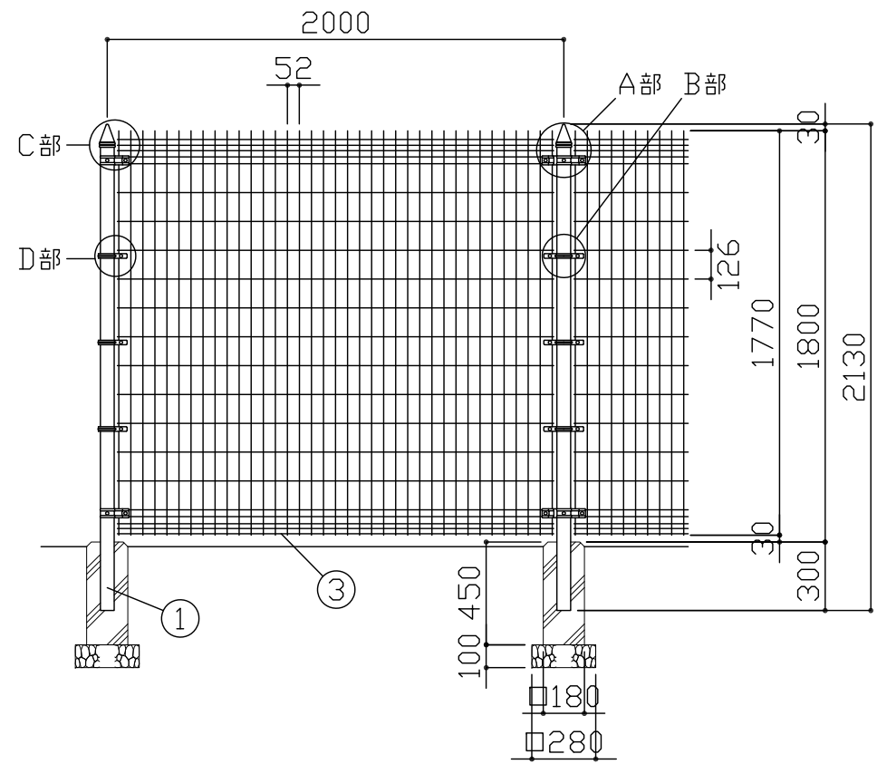
立面図 S = 1 / 30
