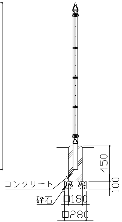
側面図 S = 1 / 30
