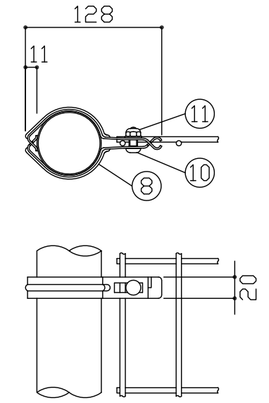
側面図 S = 1 / 20
