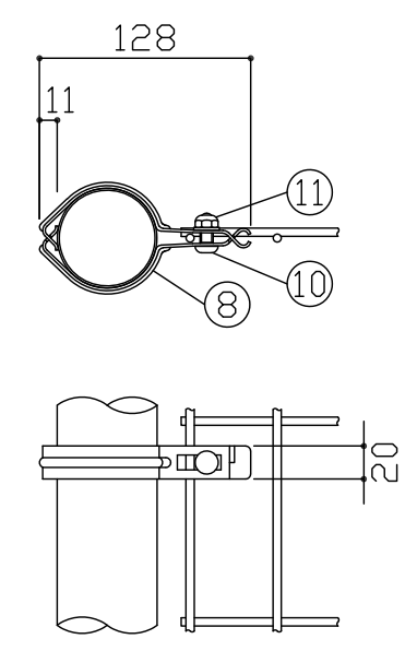
側面図 S = 1 / 20
