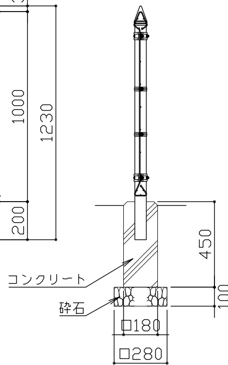
側面図 S = 1 / 20
