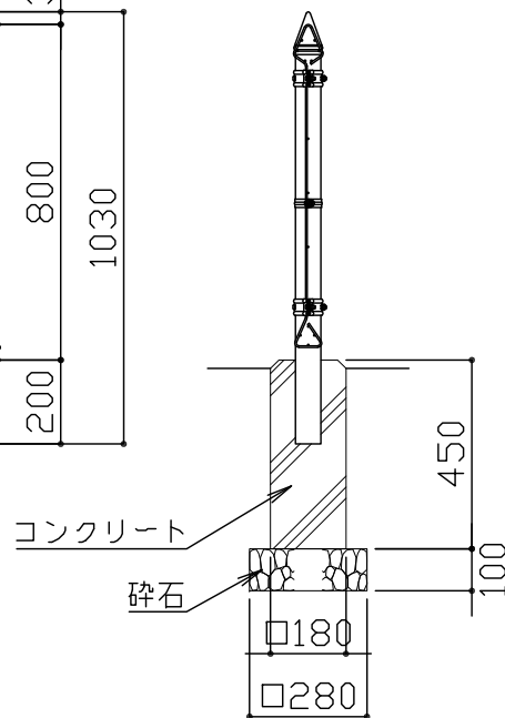
側面図 S = 1 / 20
