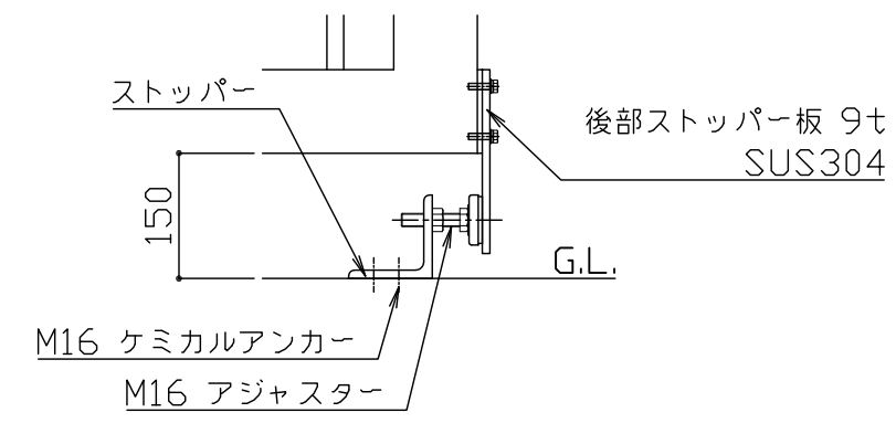
全閉時ストッパー詳細図 S = 1 / 10
