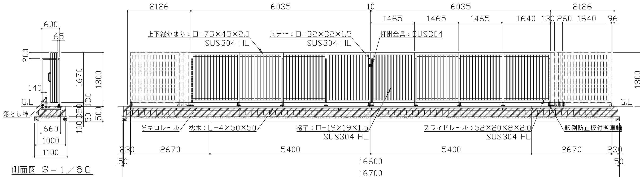
立面図 S = 1 / 60
