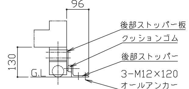
引き込み時ストッパー詳細図 S = 1 / 10
