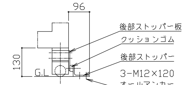
引き込み時ストッパー詳細図 S = 1 / 10
