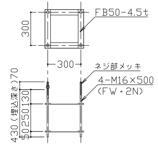
アンカーボルト詳細図 S = 1 / 20
