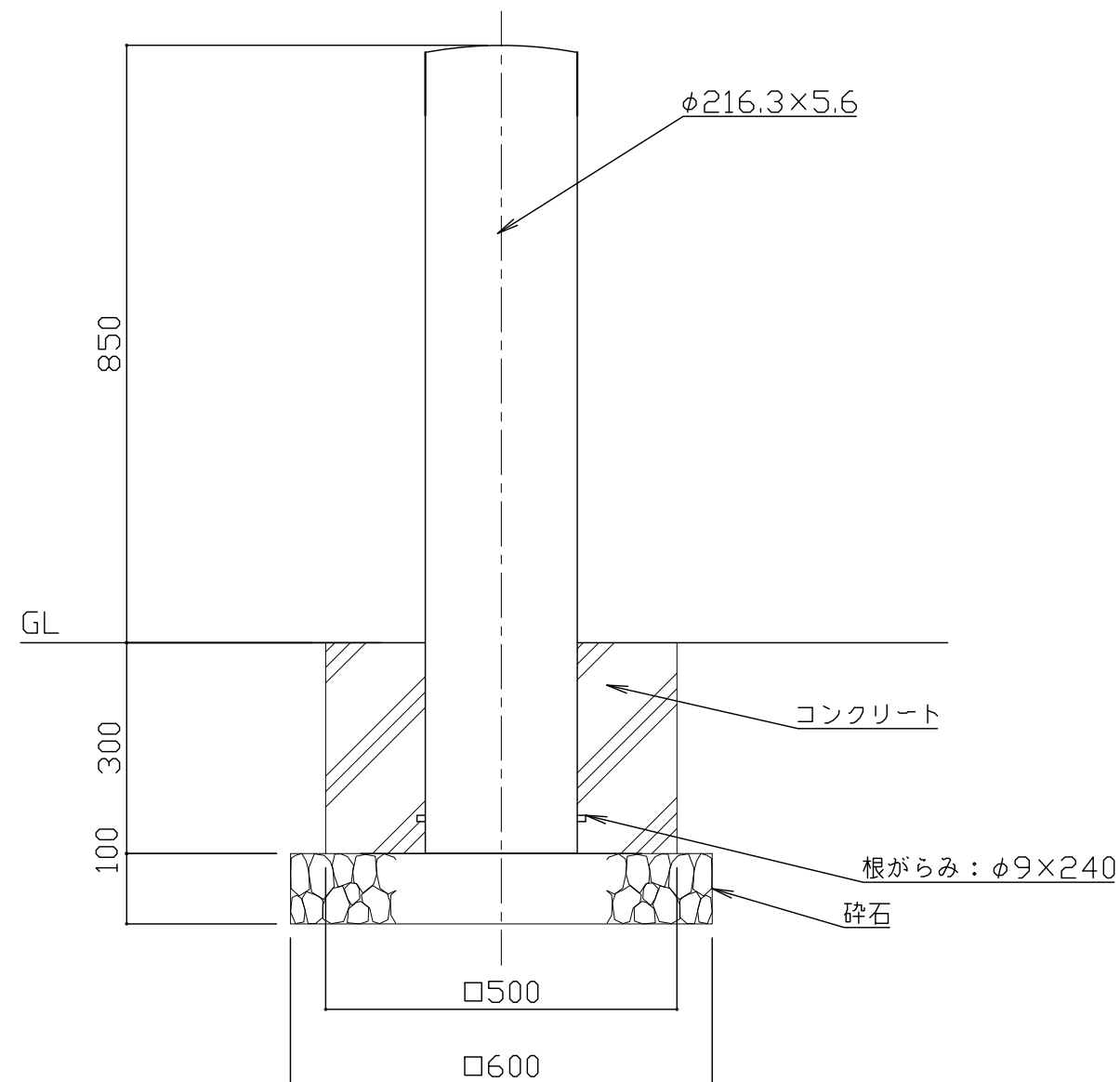
立面図 S = 1 / 10
