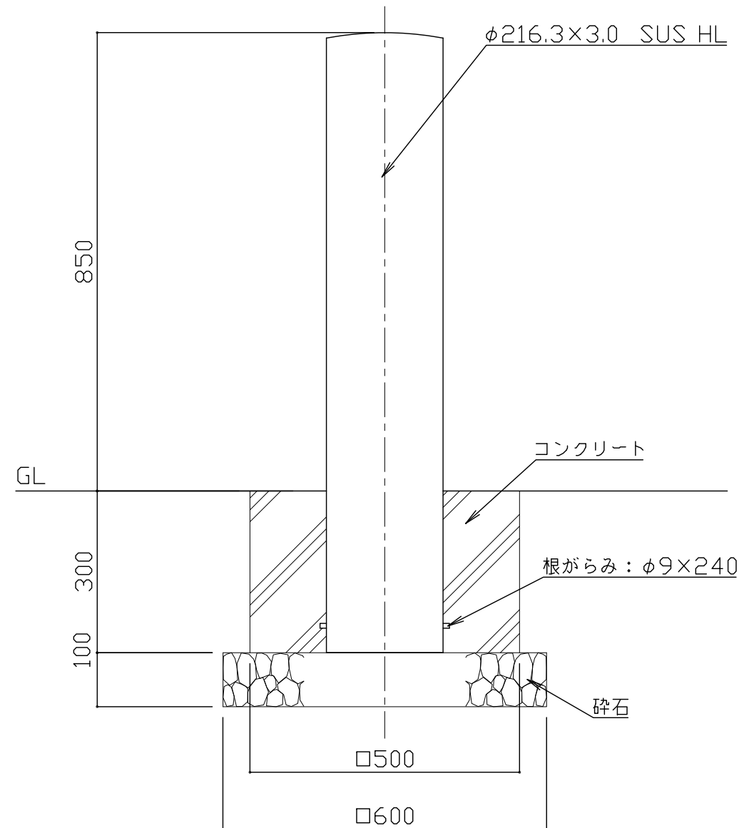
立面図 S = 1 / 10
