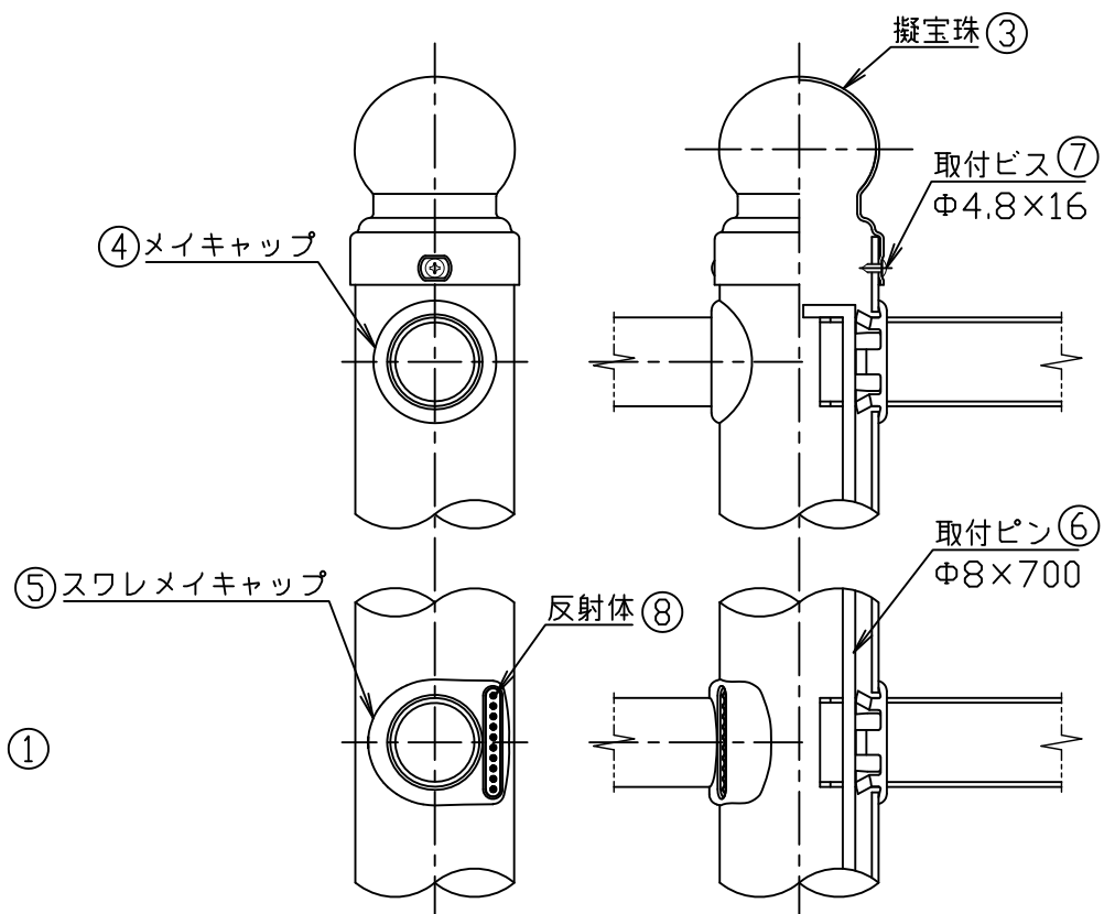
取付部詳細図 S = 1 / 4
