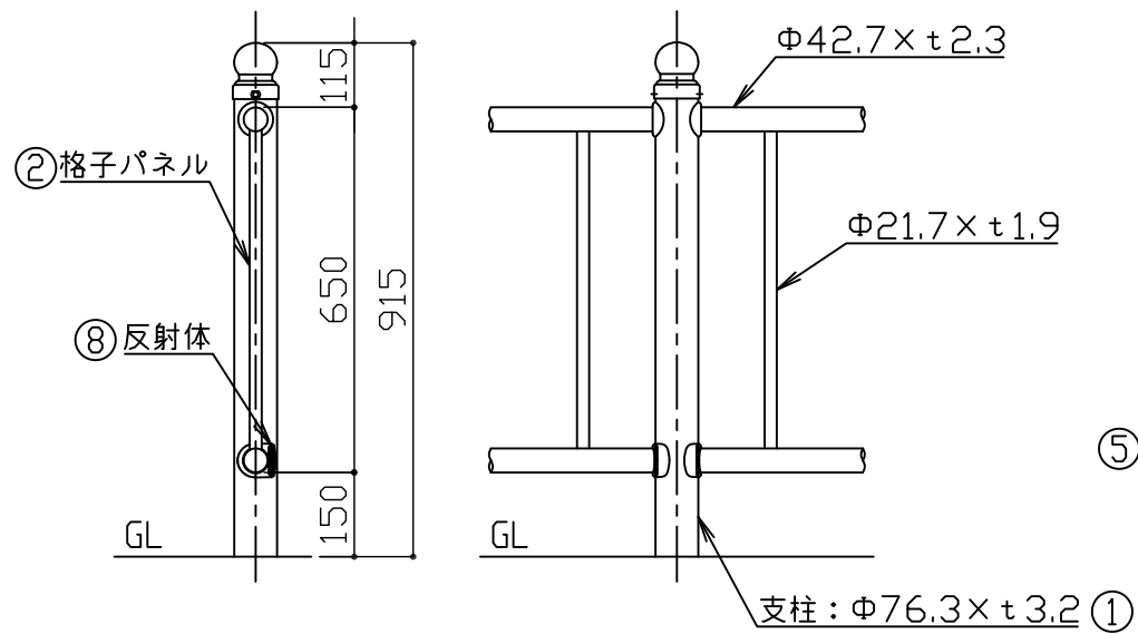
支柱図 S = 1 / 15
