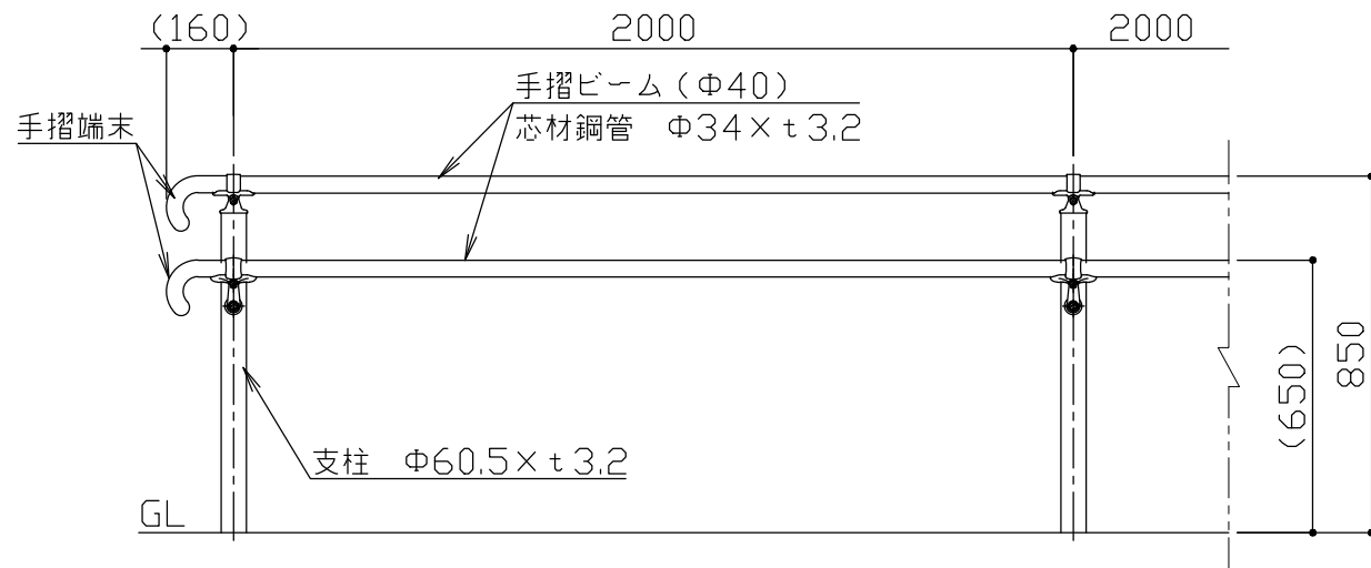
設置図 S = 1 / 20
