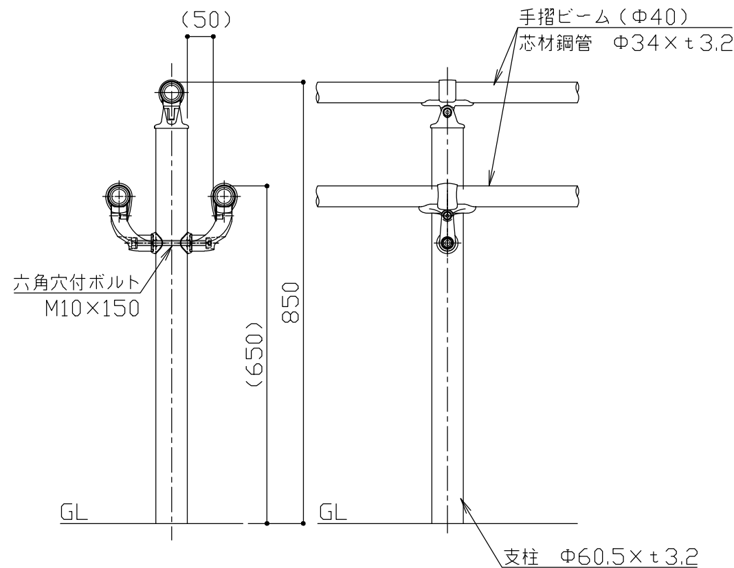
支柱図 S = 1 / 10
