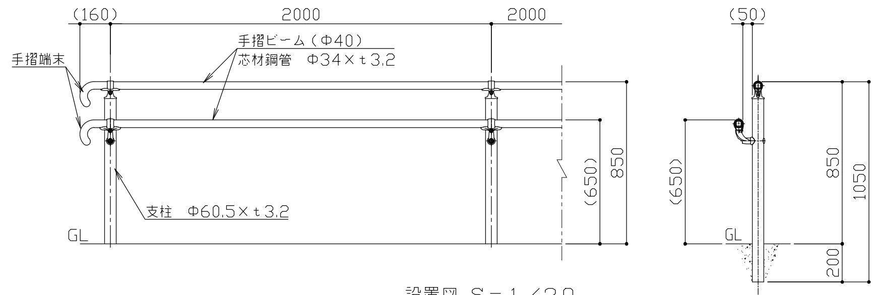
設置図 S = 1 / 20
