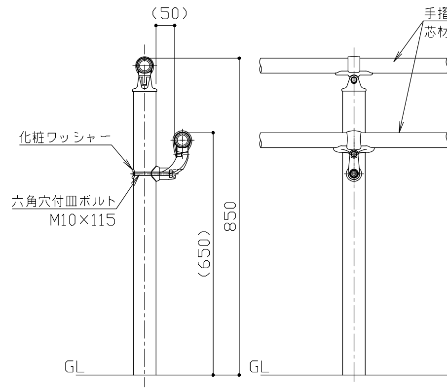
支柱図 S = 1 / 10
