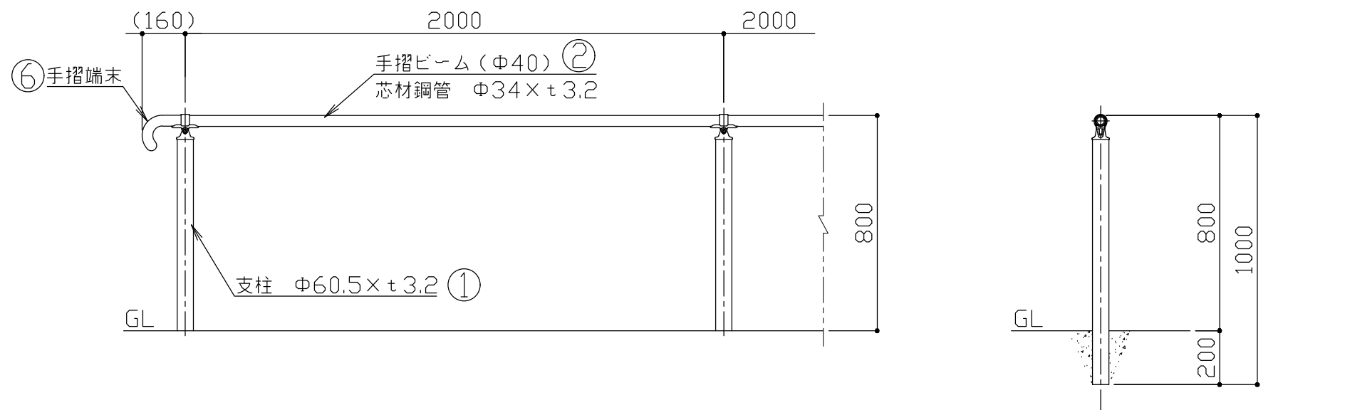
設置図 S = 1 / 2 0
