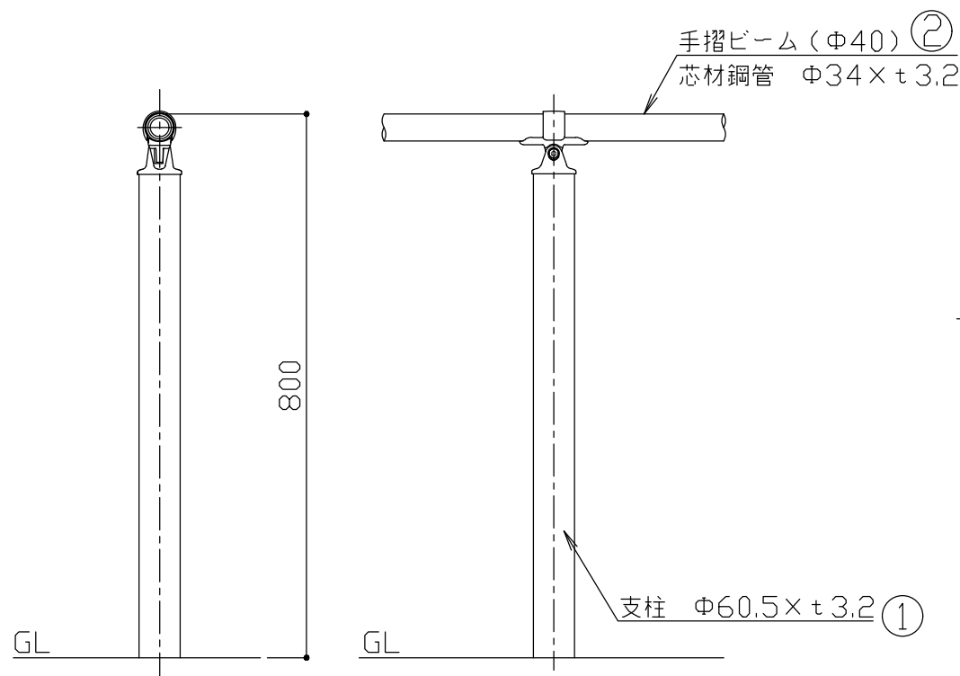
支柱図 S = 1 / 1 0
