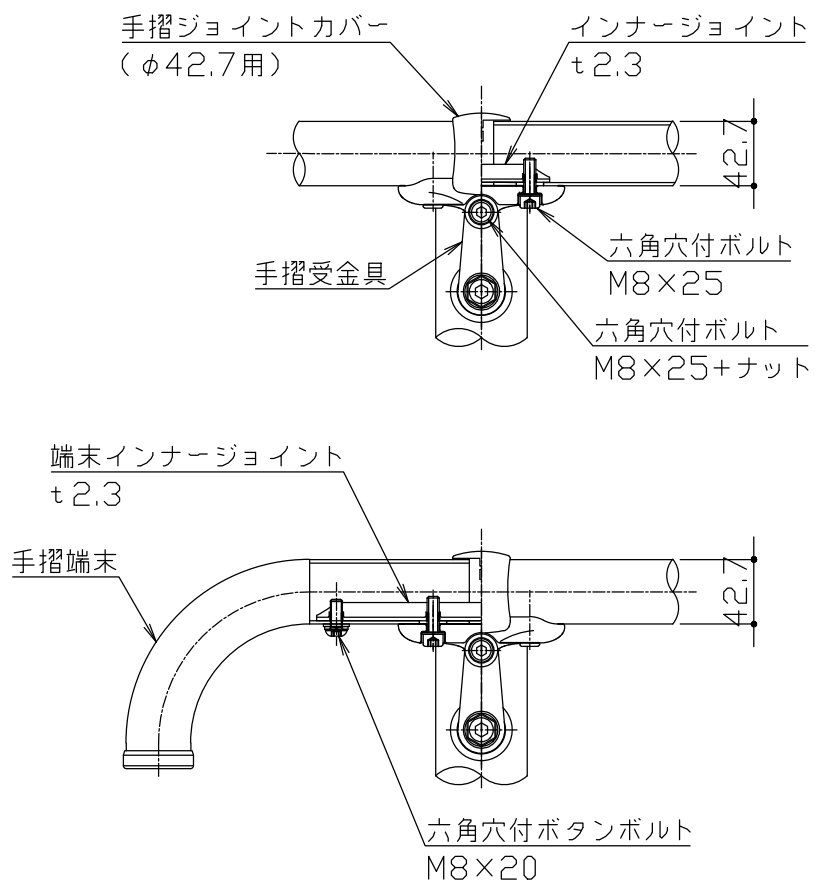
取付部詳細図 S = 1 / 5
