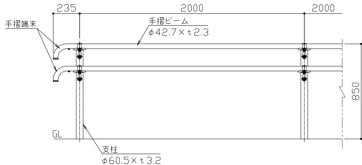
設置図 S = 1 / 2 0
