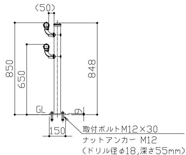
設置図 S = 1 / 2 0
