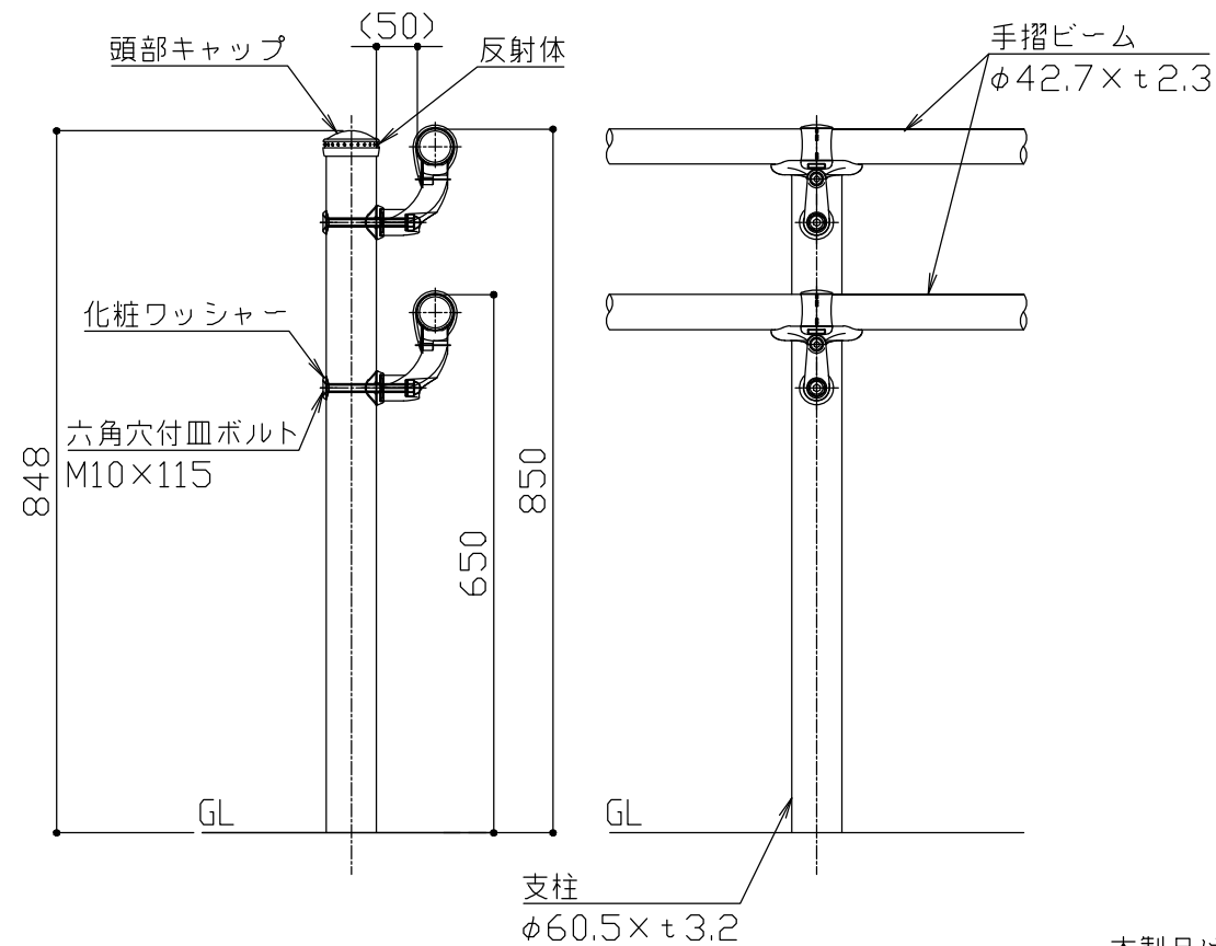
支柱図 S = 1 / 1 0
