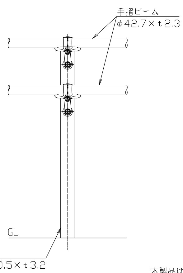
支柱図 S = 1 / 1 0
