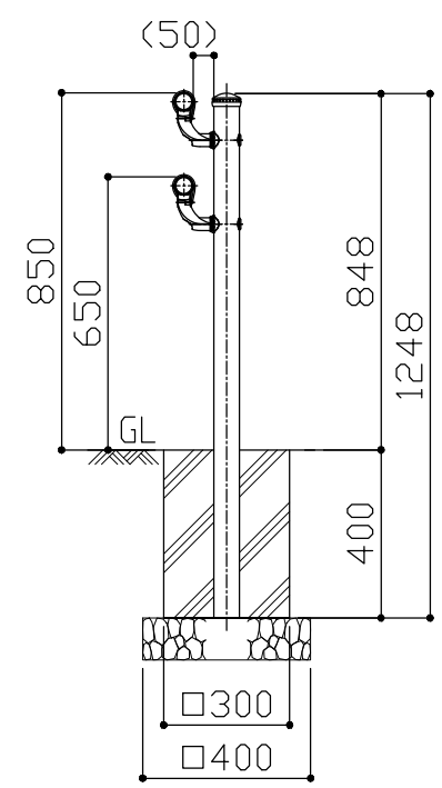
設置図 S = 1 / 2 0
