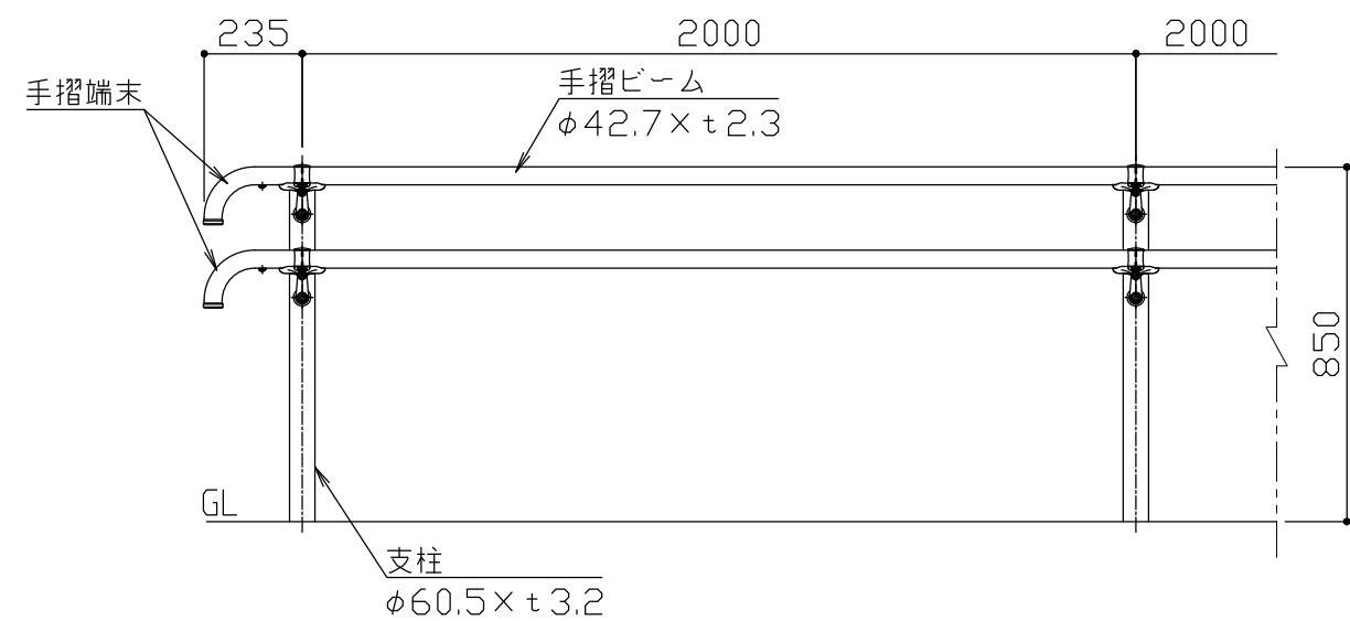
設置図 S = 1 / 2 0
