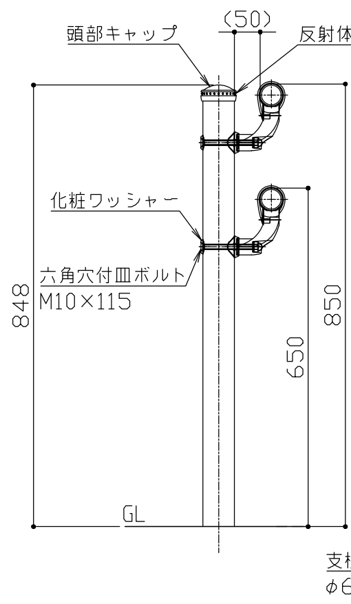
支柱図 S = 1 / 1 0
