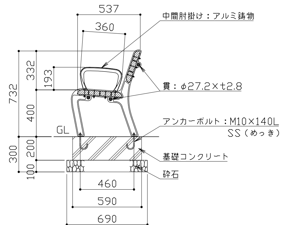
断面図 S = 1 / 20
