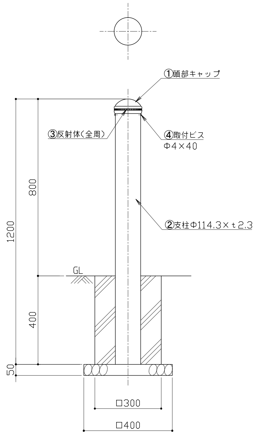
立面図 S = 1 / 1 0
