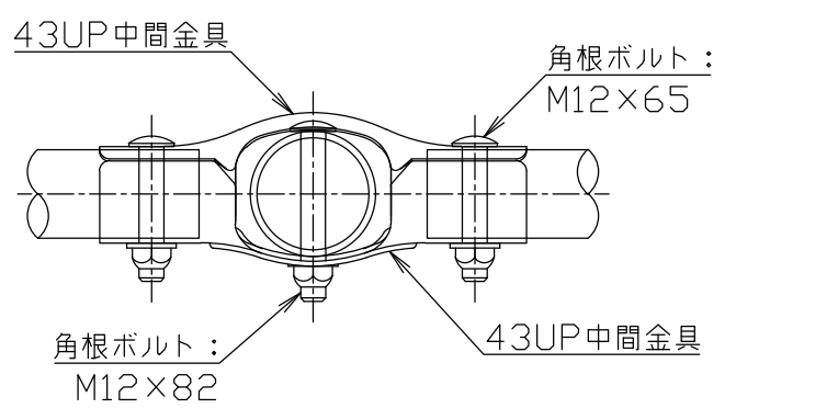
取付部詳細図 S = 1 / 4
