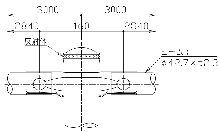
立面図 S = 1 / 20
