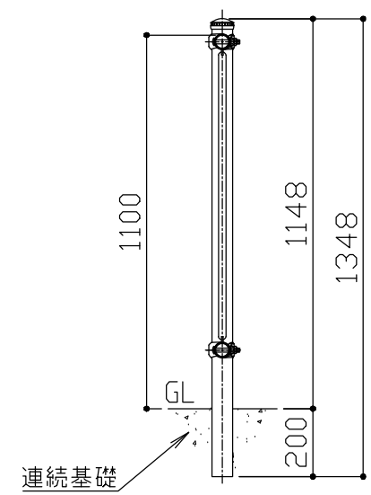
側面図 S = 1 / 20
