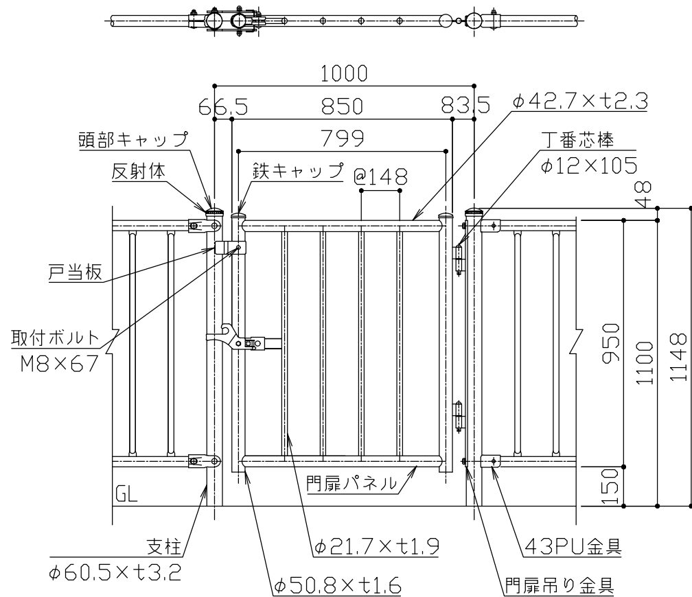
立面図 S = 1 / 20
