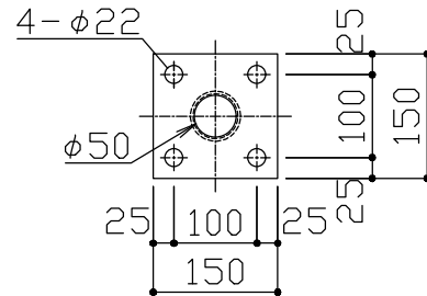
ベースプレート詳細図 S = 1 / 10
