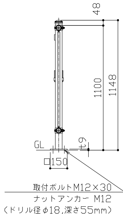
側面図 S = 1 / 20
