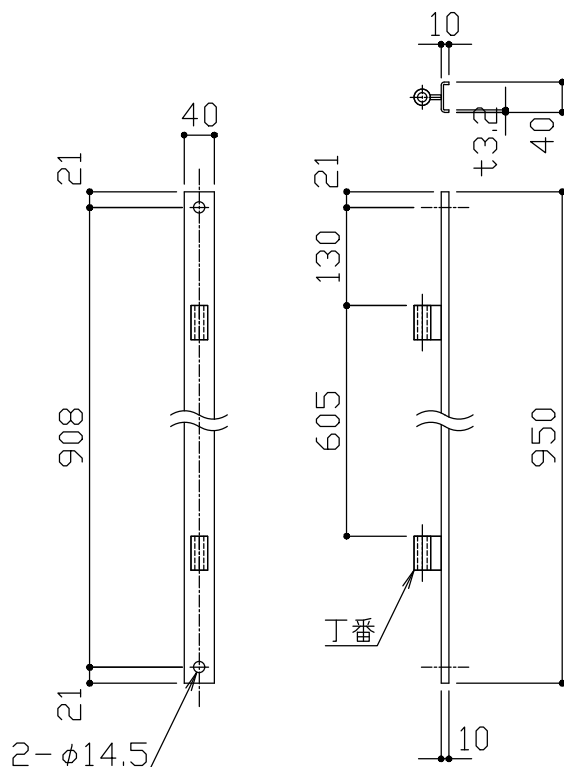
門扉吊り金具詳細図 S = 1 / 1 0
