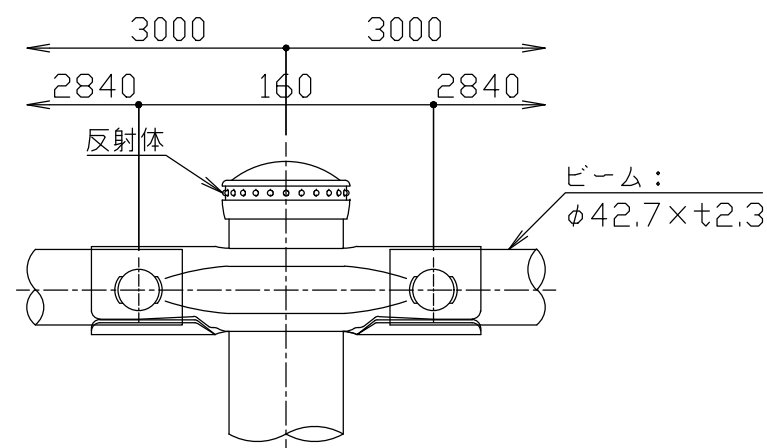
立面図 S = 1 / 20
