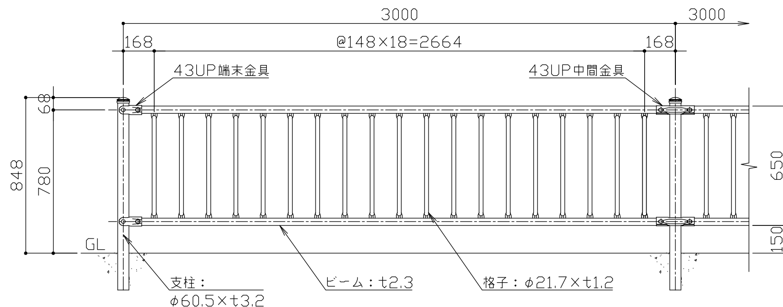
立面図 S = 1 / 20
