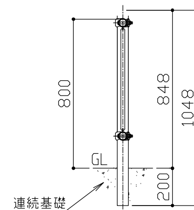
側面図 S = 1 / 20
