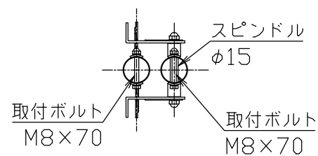
A-A断面図 S = 1 / 10
