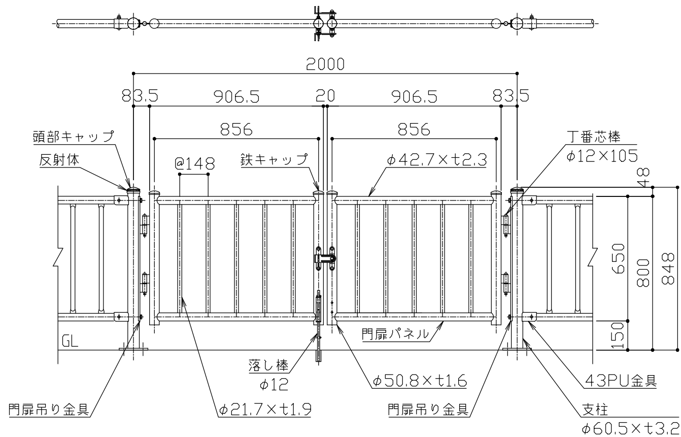
立面図 S = 1 / 20
