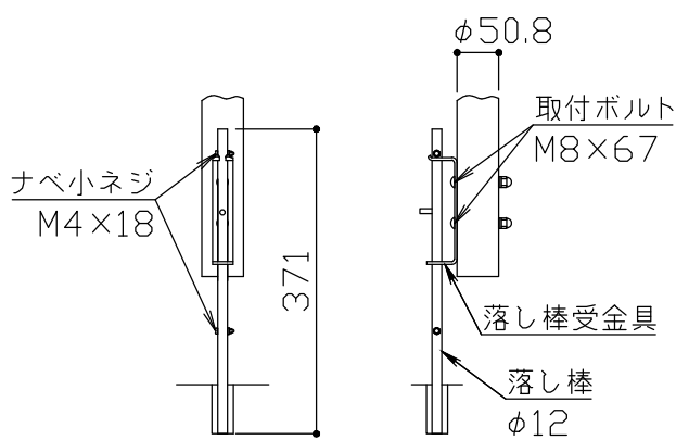
落とし棒詳細図 S = 1 / 10
