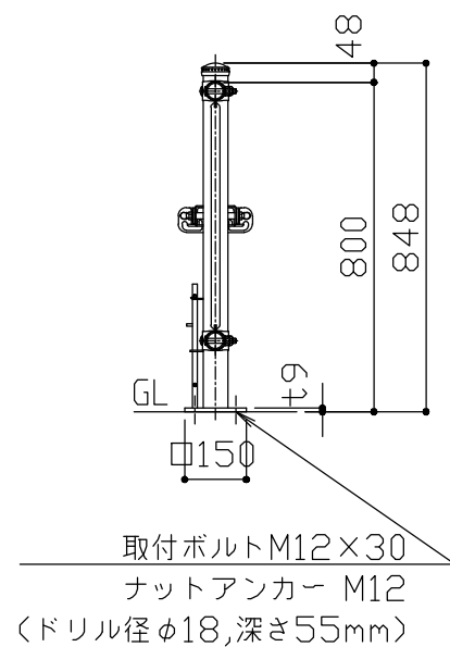
側面図 S = 1 / 20
