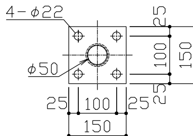
ベースプレート詳細図 S = 1 / 10
