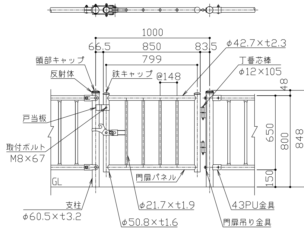
立面図 S = 1 / 20
