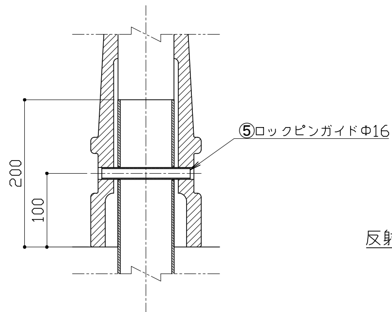
下部断面詳細図 S = 1 / 5
