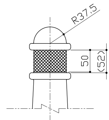
反射シート貼付部詳細図 S = 1 / 5
