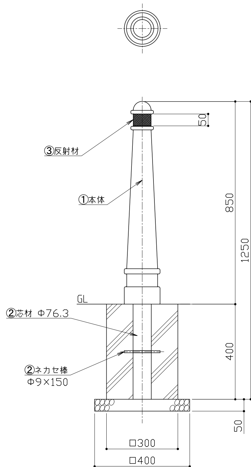
立面図 S = 1 / 10
