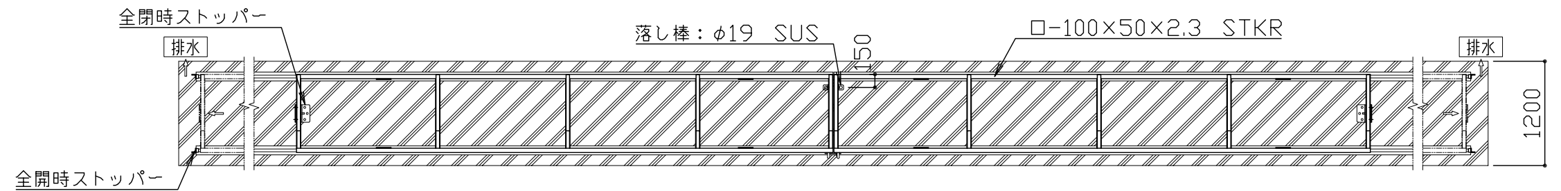
平面图 S = 1 / 60
