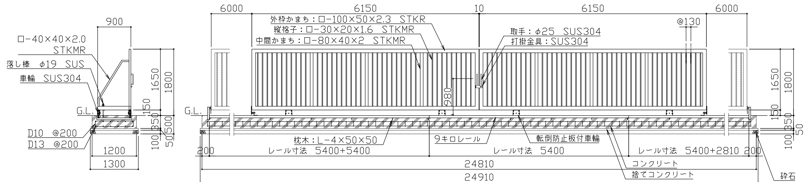
立面図 S = 1 / 60
