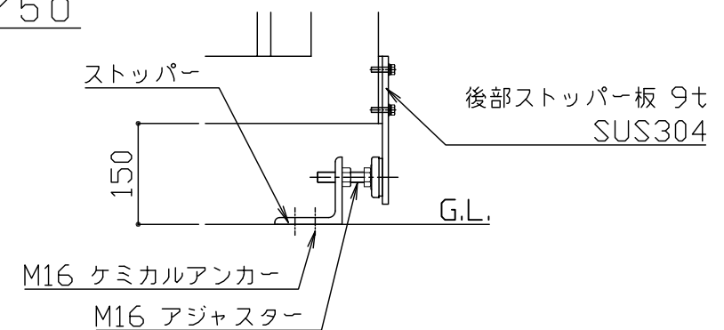
全開時ストッパー詳細図 S = 1 / 10
