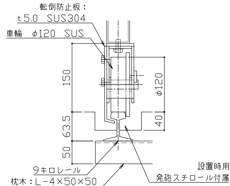
車輪部詳細図 S = 1 / 5
