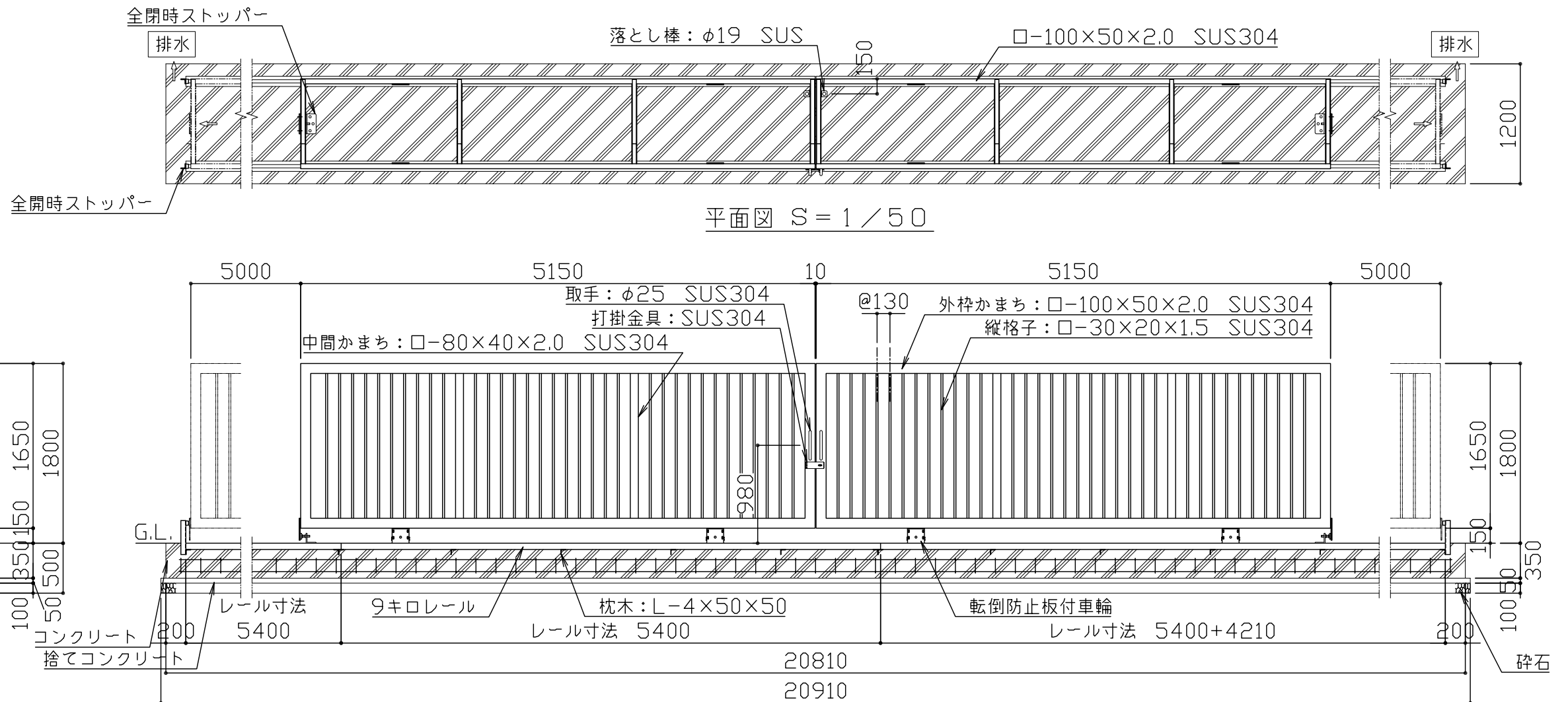
立面図 S = 1 / 50
