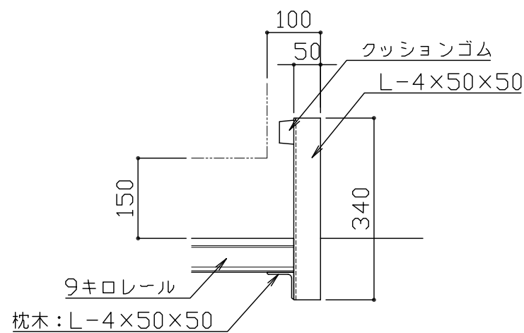
全開時ストッパー詳細図 S = 1 / 10
