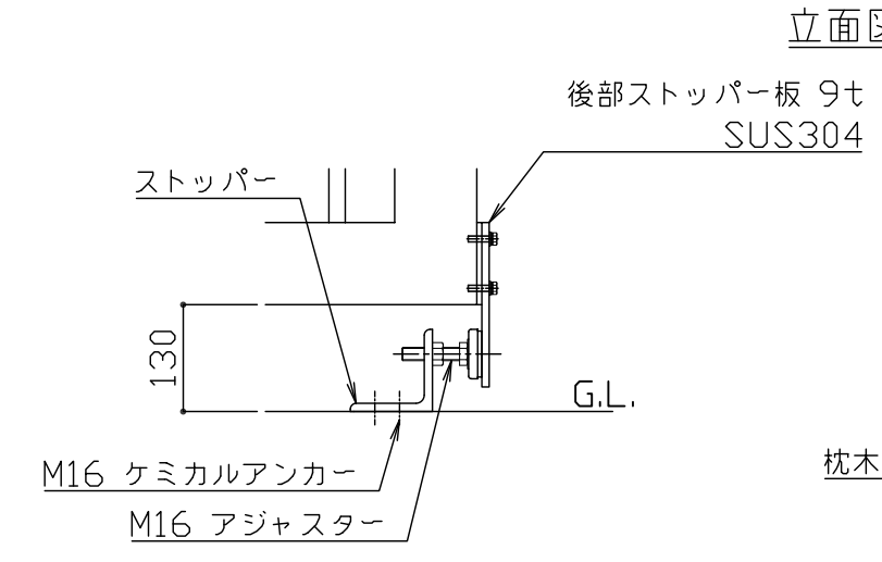
全閉時ストッパー詳細図 S = 1 / 10
