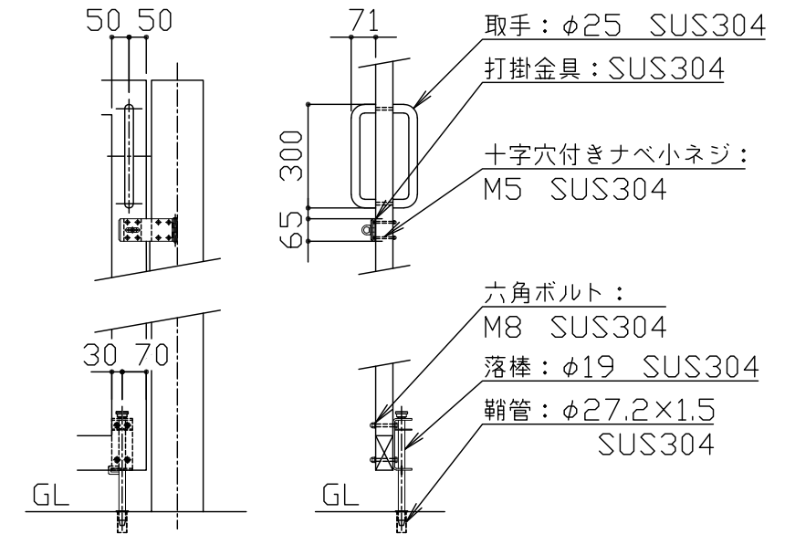
詳細図 S = 1 / 15
