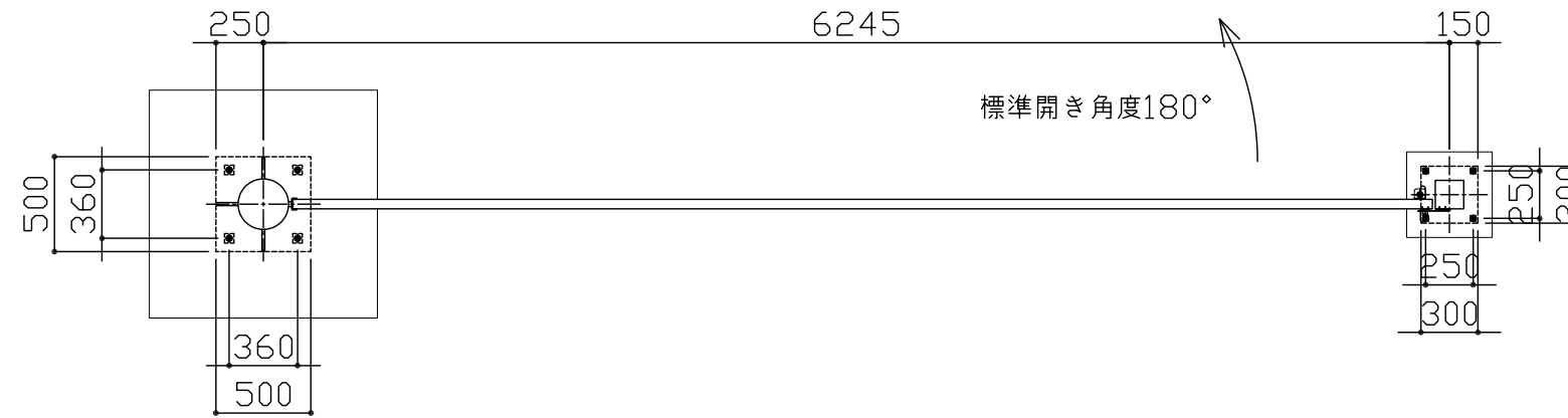
平面図 S = 1 / 40
