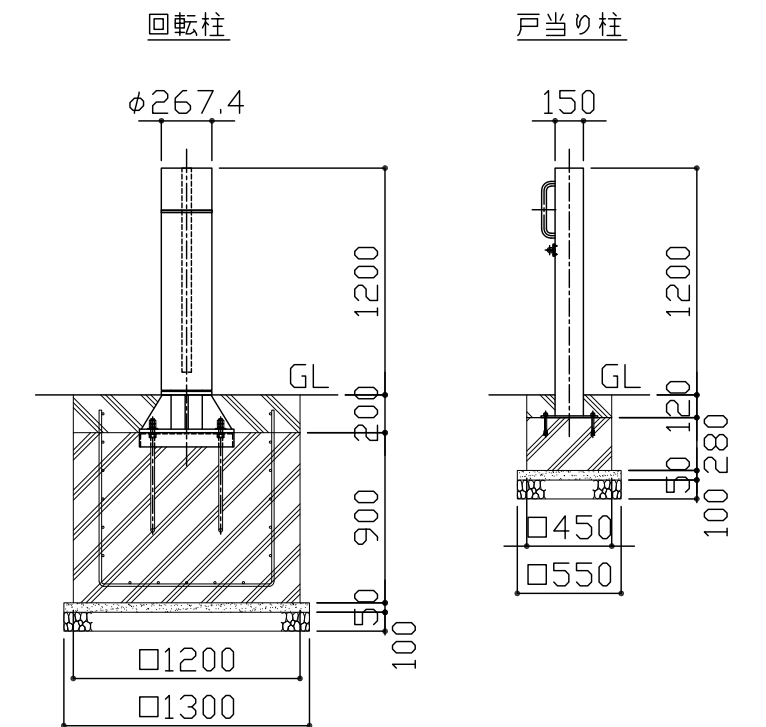
側面図 S = 1 / 40
