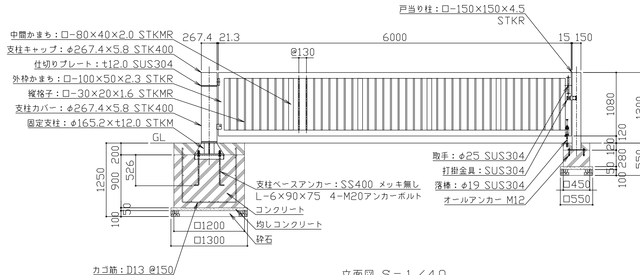
立面图 S = 1 / 40
