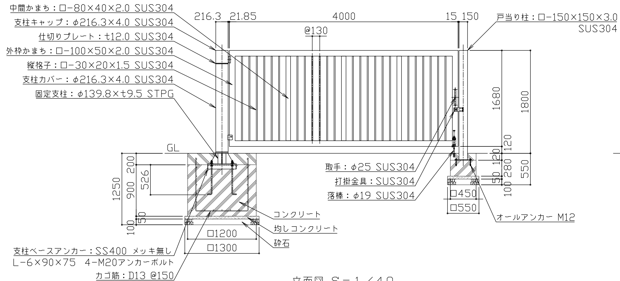
立面図 S = 1 / 40
