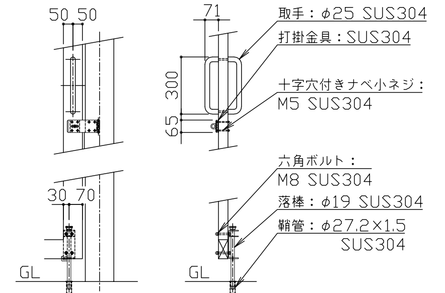
詳細図 S = 1 / 15
