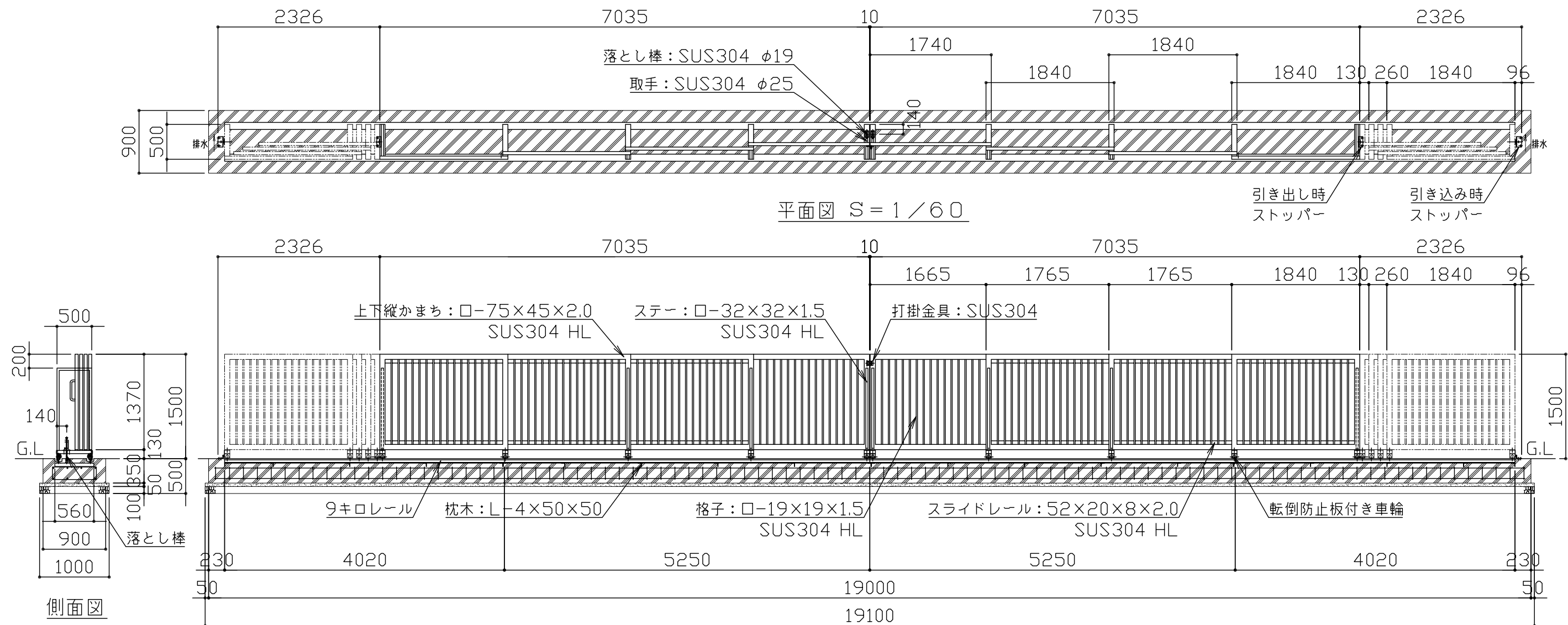
立面図 S = 1 / 6 0
