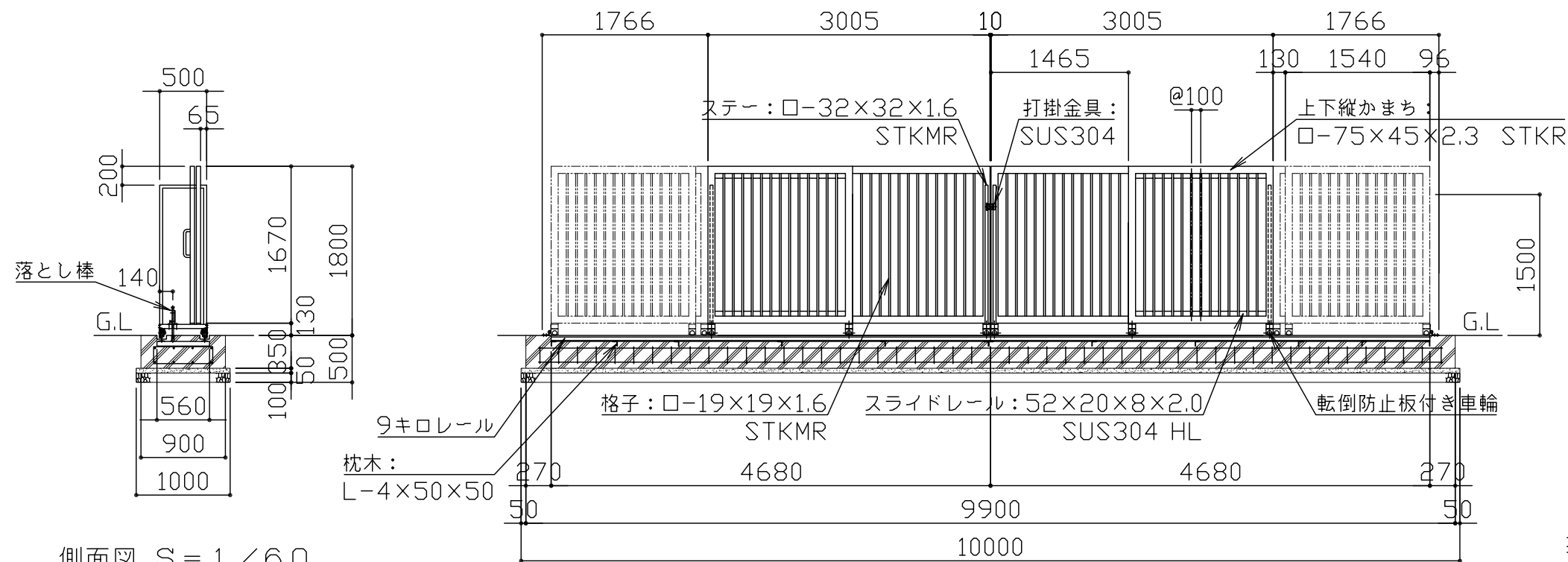
側面図 S = 1 / 60
