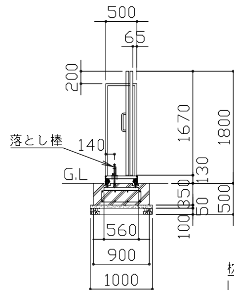
側面図 S = 1 / 60
