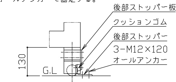
引き出し時ストッパー詳細図 S = 1 / 1 0
