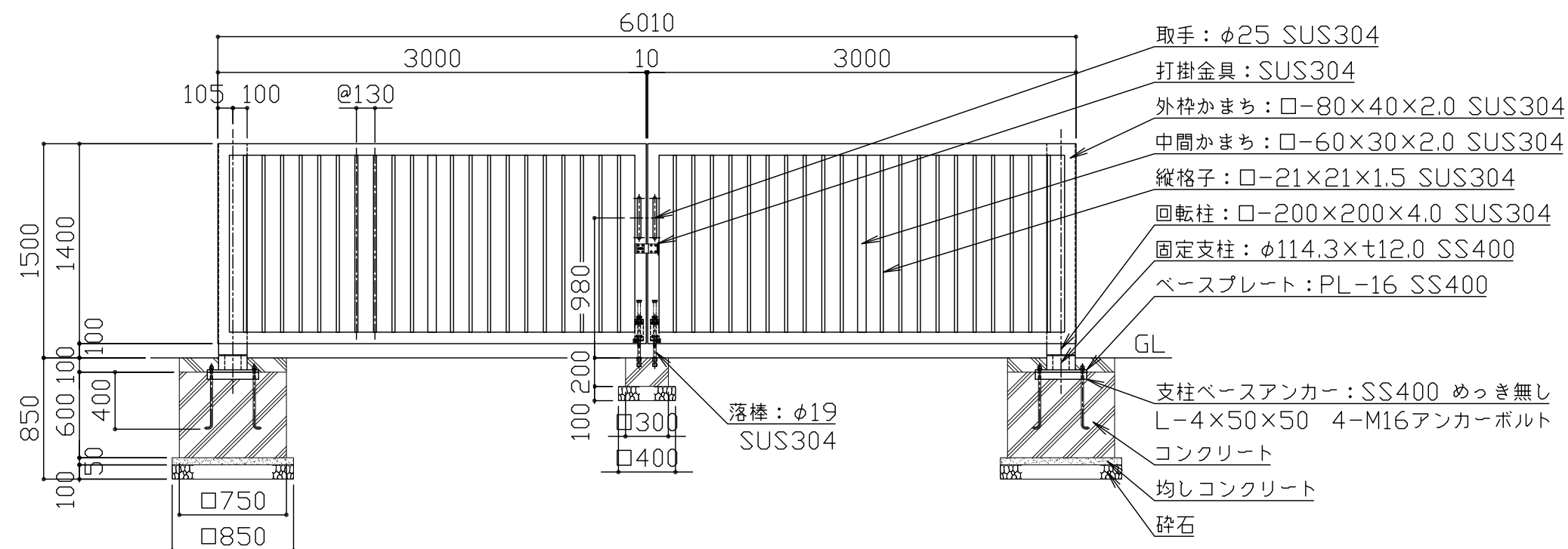
立面图 S = 1 / 40
