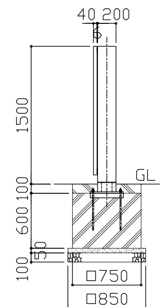
側面図 S = 1 / 40
