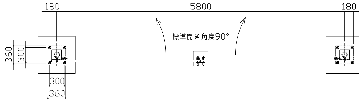
平面图 S = 1 / 40
