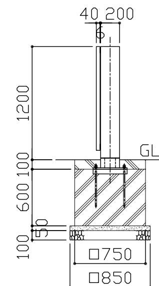
側面図 S = 1 / 40
