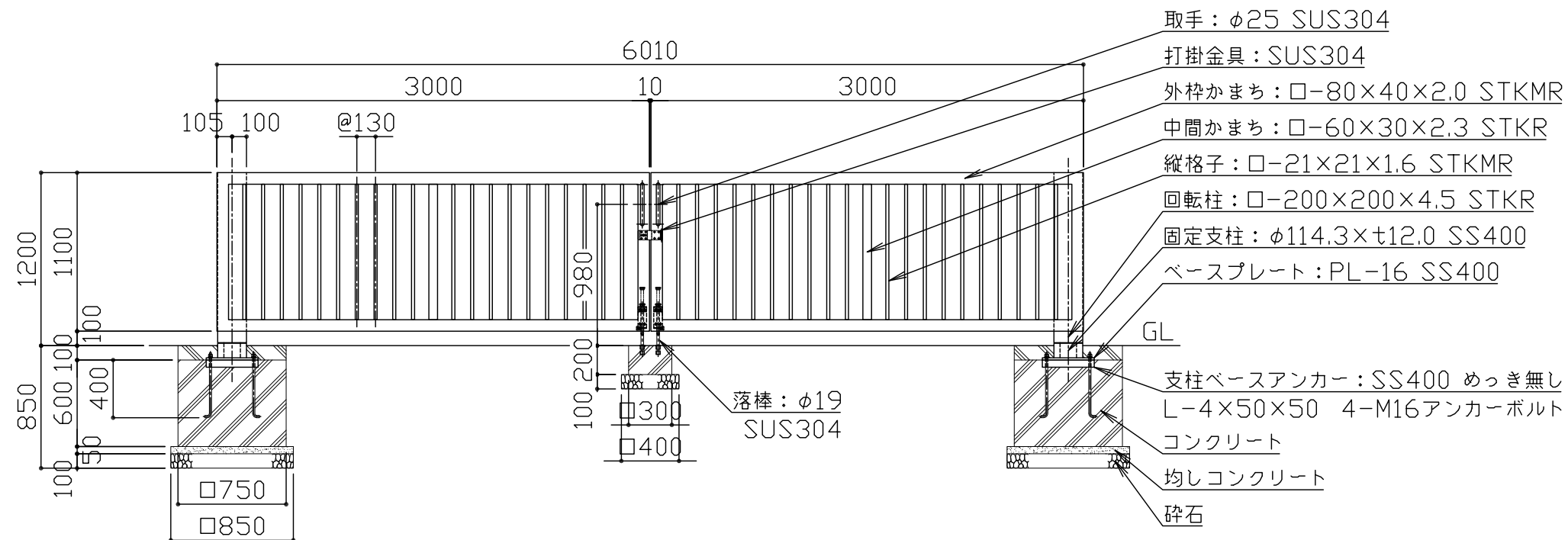
立面图 S = 1/40
