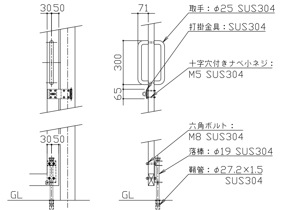
詳細図 S = 1 / 1 5
