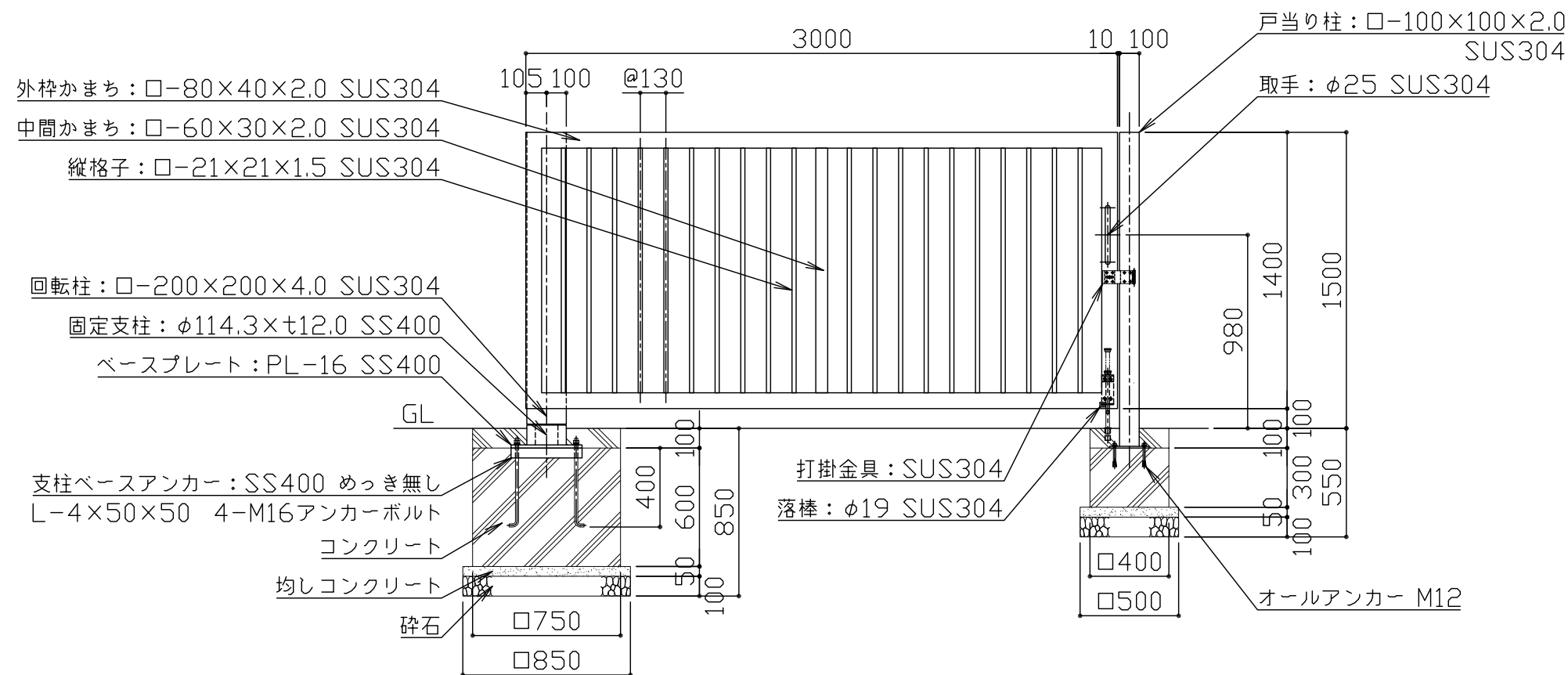
立面图 S = 1 / 30
