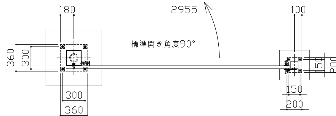
平面図 S = 1 / 30
