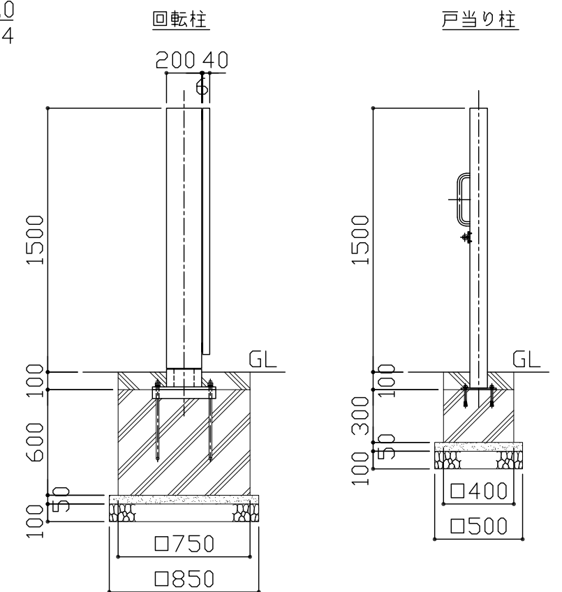
側面図 S = 1 / 30
