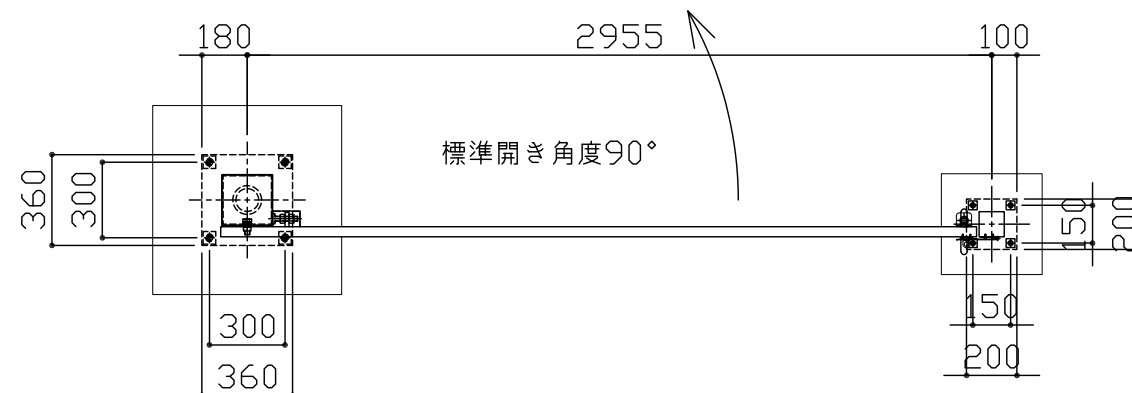
平面図 S = 1/30
