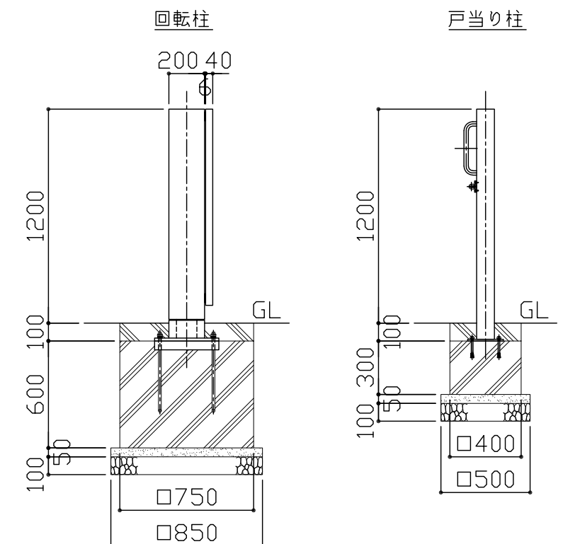
側面図 S = 1 / 30
