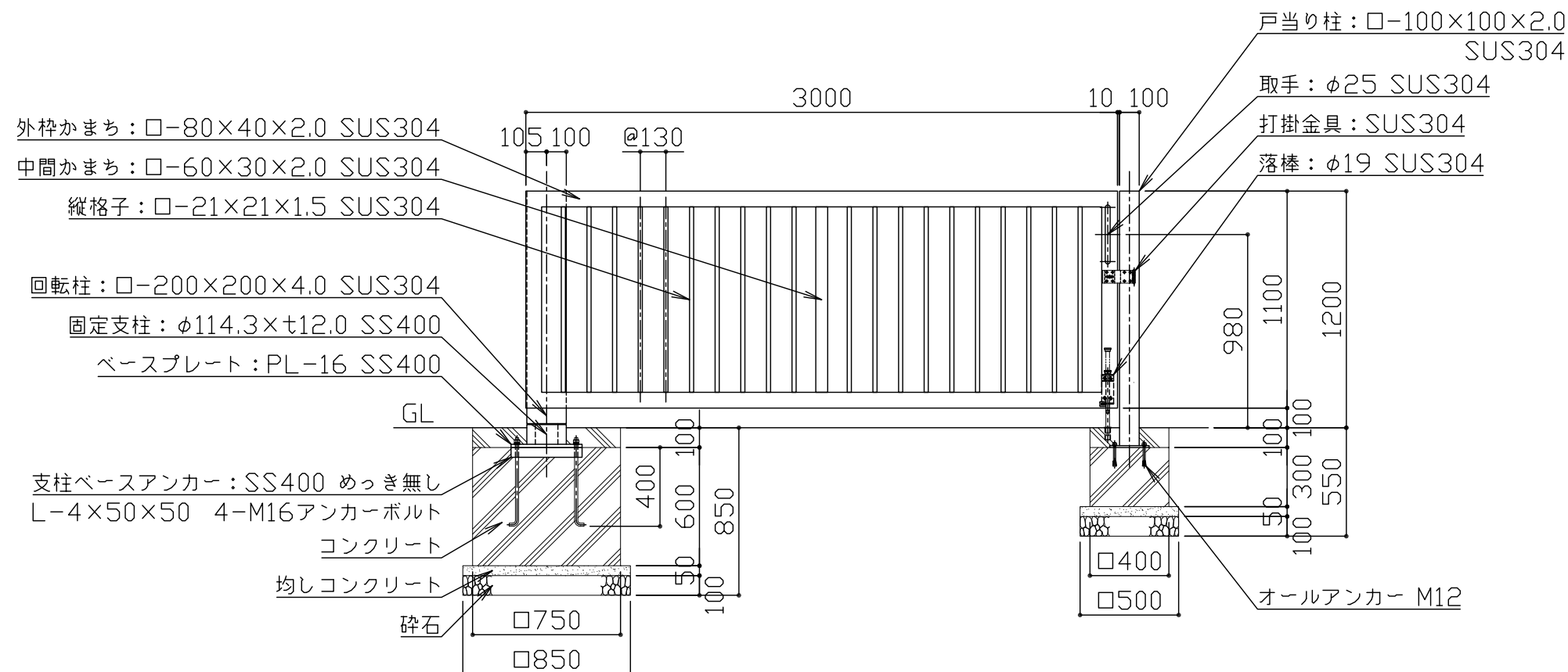
立面图 S = 1 / 30
