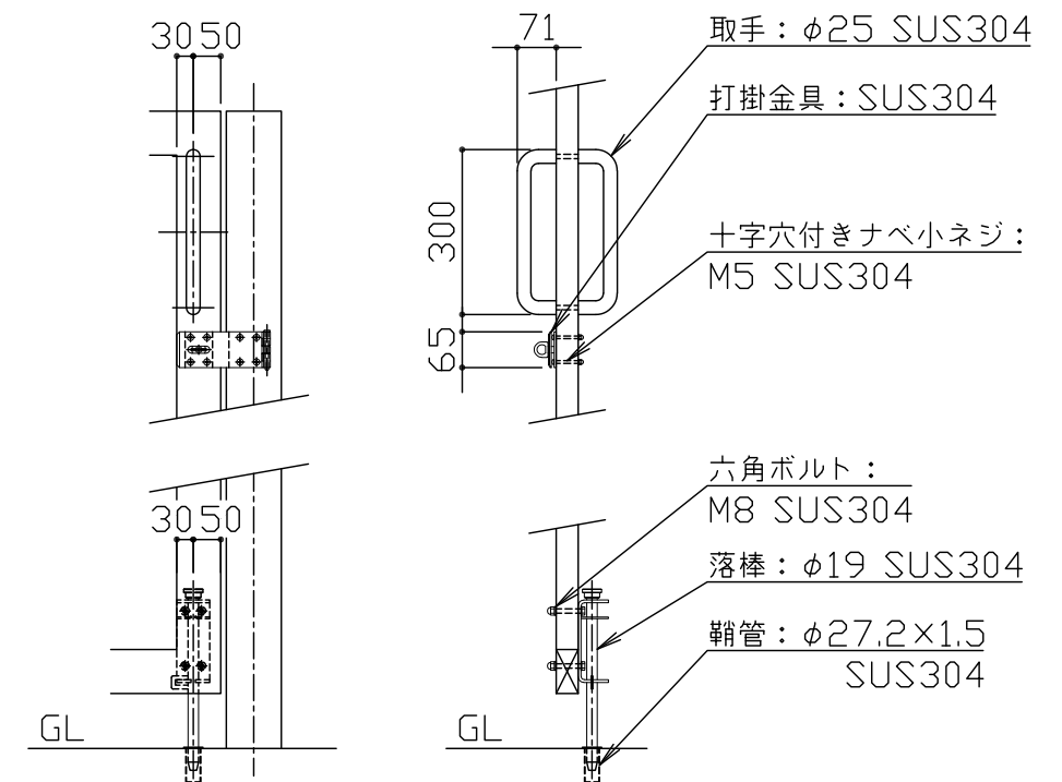
詳細図 S = 1 / 1 5
