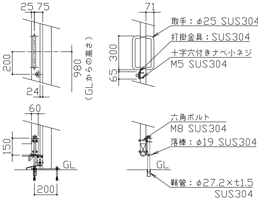
詳細図 S = 1 / 20
