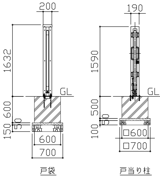
側面図 S = 1 / 50
