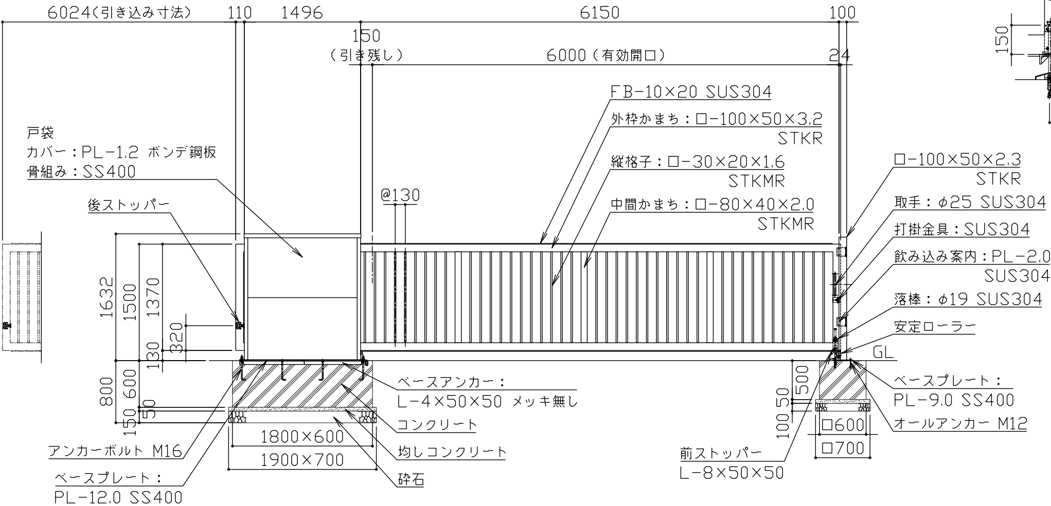
立面図 S = 1 / 50
