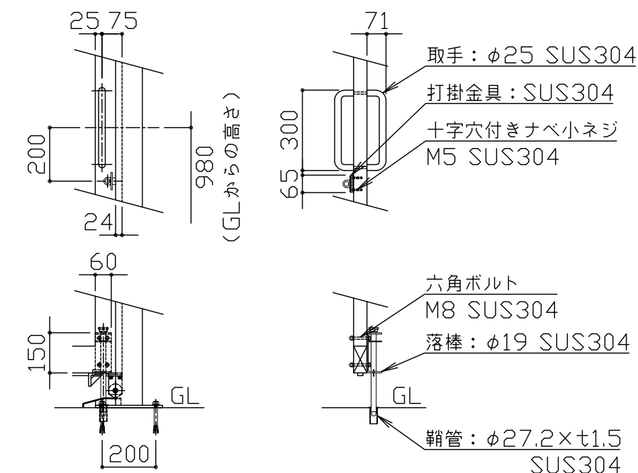
詳細図 S = 1 / 20
