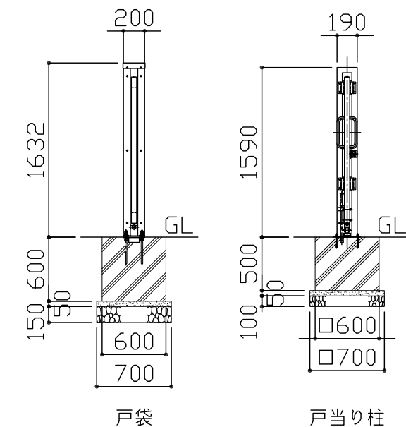
側面図 S = 1 / 50
