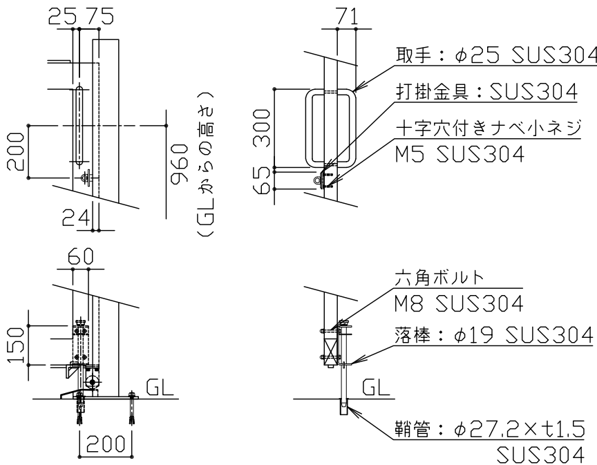
詳細図 S = 1 / 20
