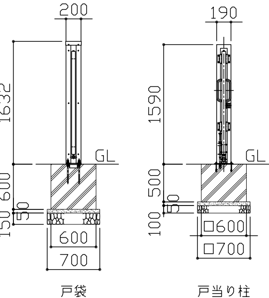
側面図 S = 1 / 50
