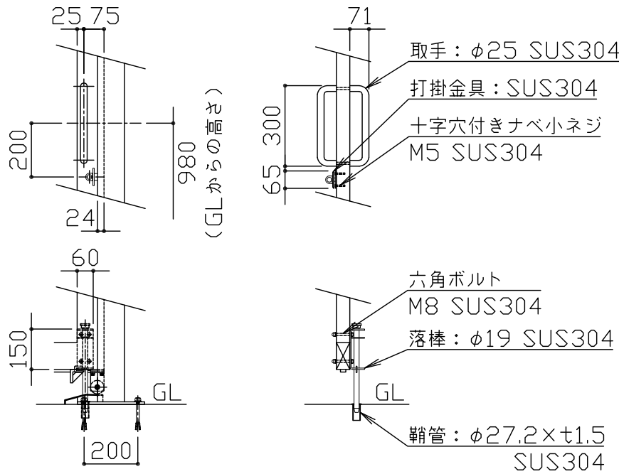
詳細図 S = 1 / 20
